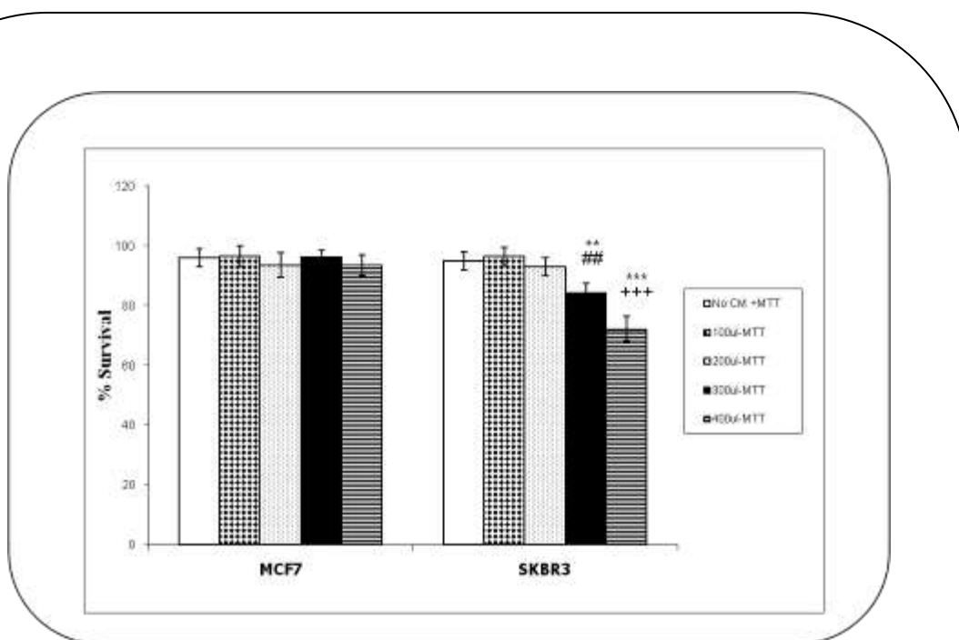
شکل ۹- دیاگرام مربوط به نتایج MTT
