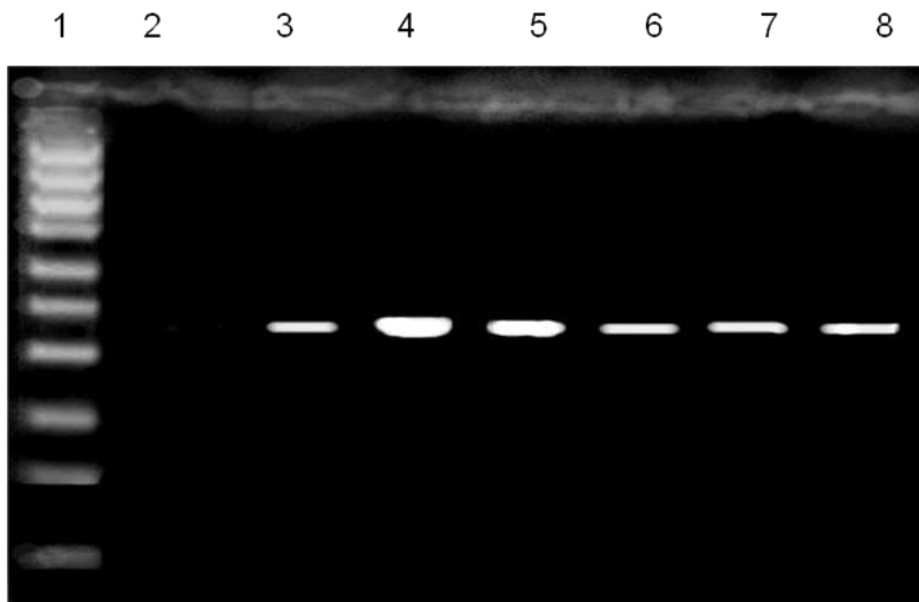
شکل ۱۰- RT-PCR برای بررسی بیان گیرنده HER2 در سلول های تحت تیمار با هرسپتین. ۱. 100bp DNA ladder، ۲. کنترل منفی ۳. 293T H، ۴. SKBR3، ۵. MCF7، ۶. 293T H، ۷. SKBR3 H، ۸. MCF7 H. Herceptin H.
