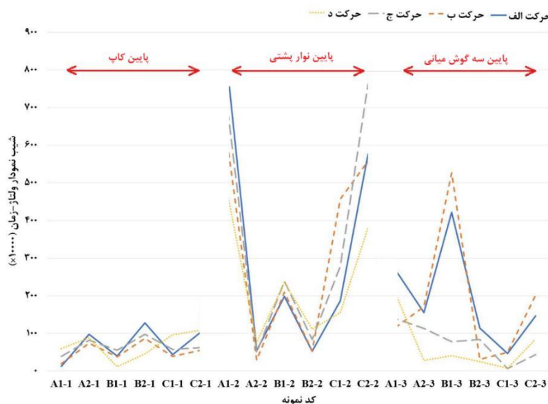
شکل ۴: مقادیر شیب نمودار ولتاژ-زمان ( \times 10000 ) در حین انجام حرکات مختلف
